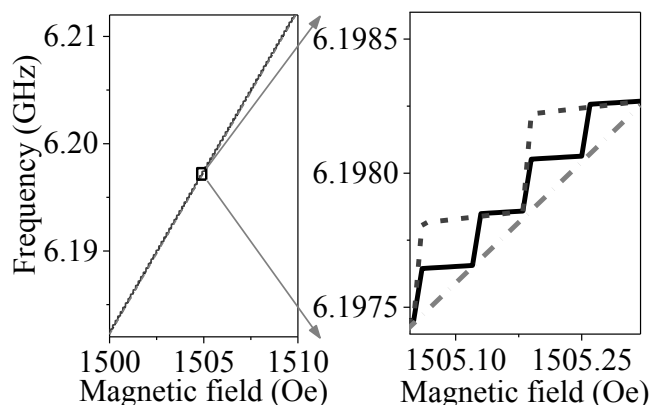
Рисунок 3. Магнитная перестройка частоты генерации в ОЭГ на оптоволоконном кабеле l_{opt} = 1000 м (сплошная линия), на оптоволоконном кабеле l_{opt} = 500 м (пунктирная линия) и на спин-волновой ЛЗ (штрих-пунктирная линия).
