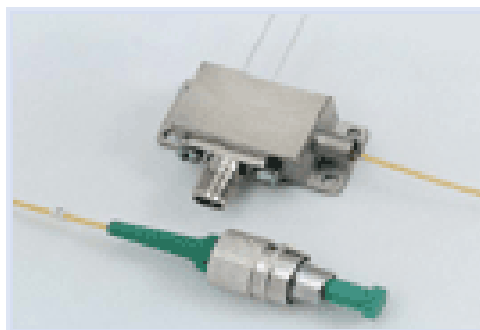
Рис. 9. Инфракрасный высокочастотный фотодиодный модуль ИФПМ 1-10 с рабочим диапазоном оптического излучения 1200 – 1620 нм (изготовитель: ОАО «Научно-производственное предприятие «Инжект», г. Саратов)
