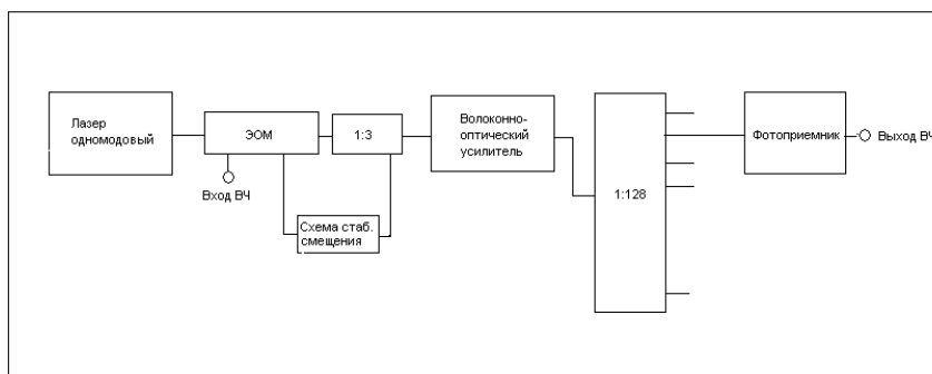
Рис.13. Блок-схема аналоговой линии. ЭОМ – электронно-оптический модулятор, 1:3 – оптический ответвитель 30%, 1:128 – оптический разветвитель на 128 каналов
