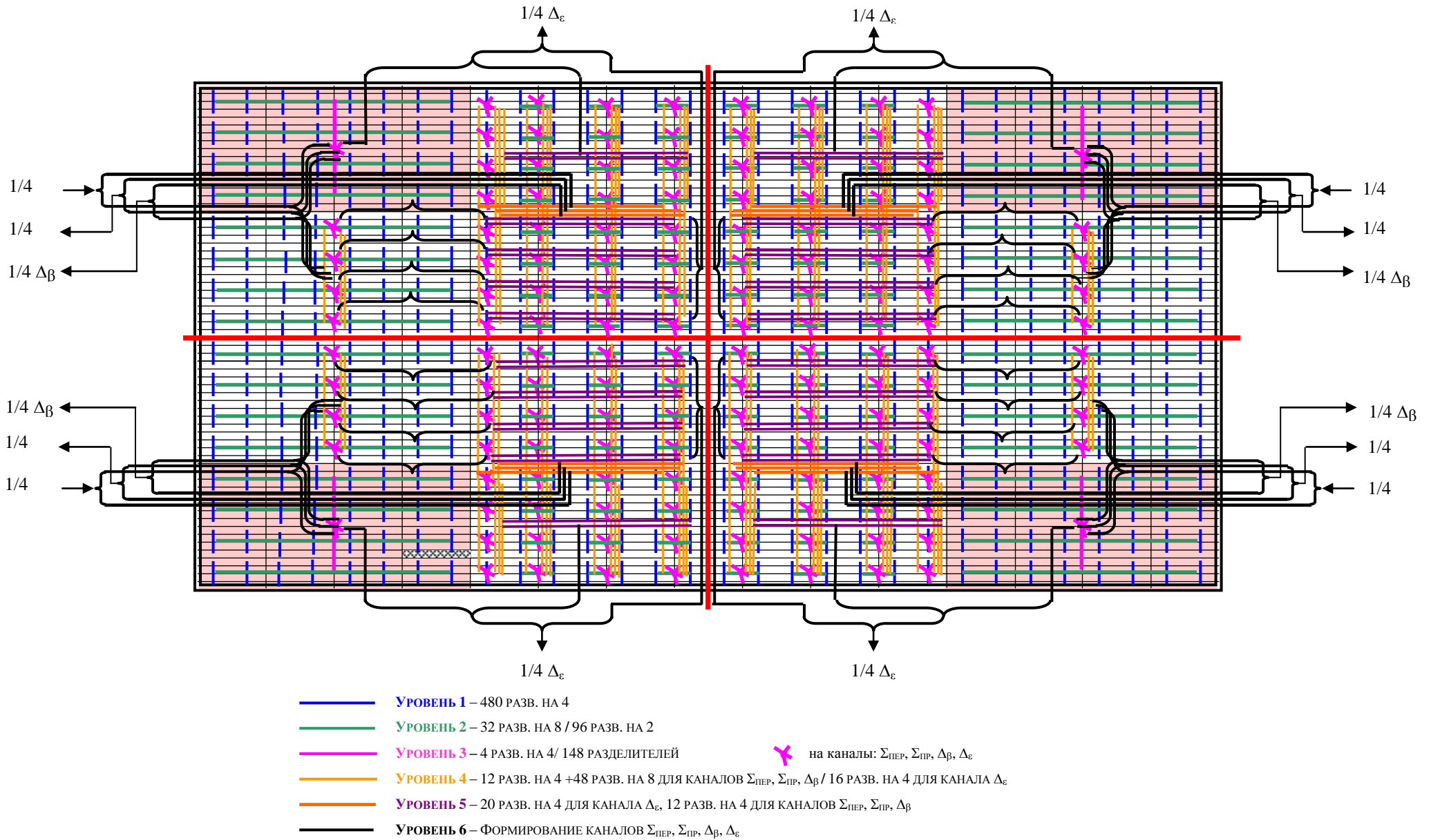
Рис. 12. Схема СВЧ разводки АФАР (эту схему, выполненную в цвете, можно посмотреть на сайте журнала)
